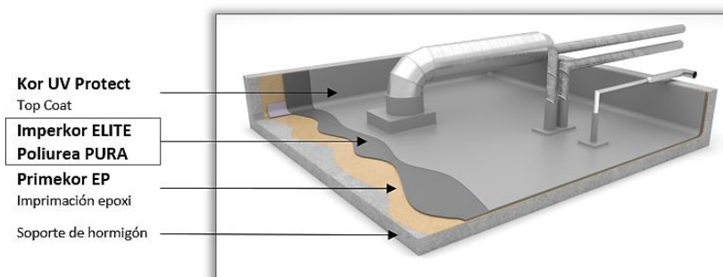
* Cubierta técnica impermeabilizada con membrana de poliurea pura Imperkor ELITE
